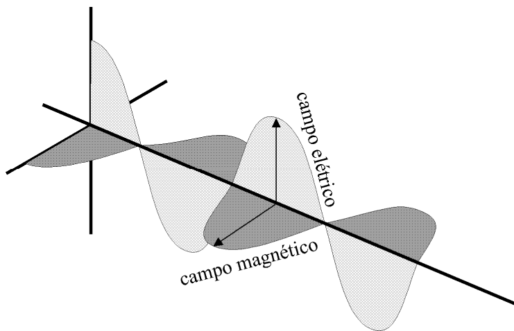
Figura 3. Representação esquemática de uma onda eletromagnética.
