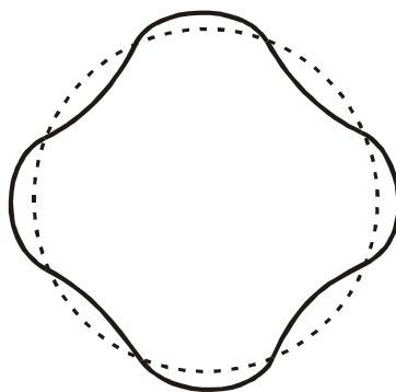
Figura 14. Representação do elétron na órbita atômica. A linha tracejada segundo o átomo de Bhor e a linha cheia segundo de Broglie.
