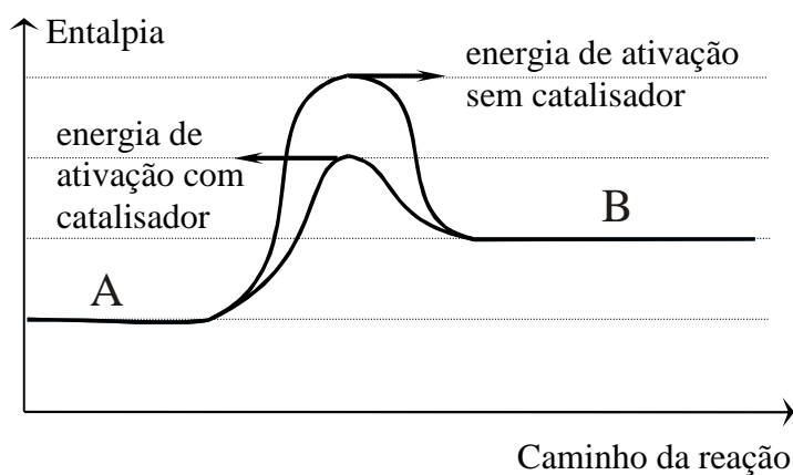
Figura 6. Representação de uma reação hipotética da substância A formando a substância B .
