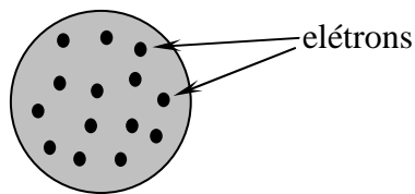
Figura 12. Representação do átomo como concebido por Thomson.
