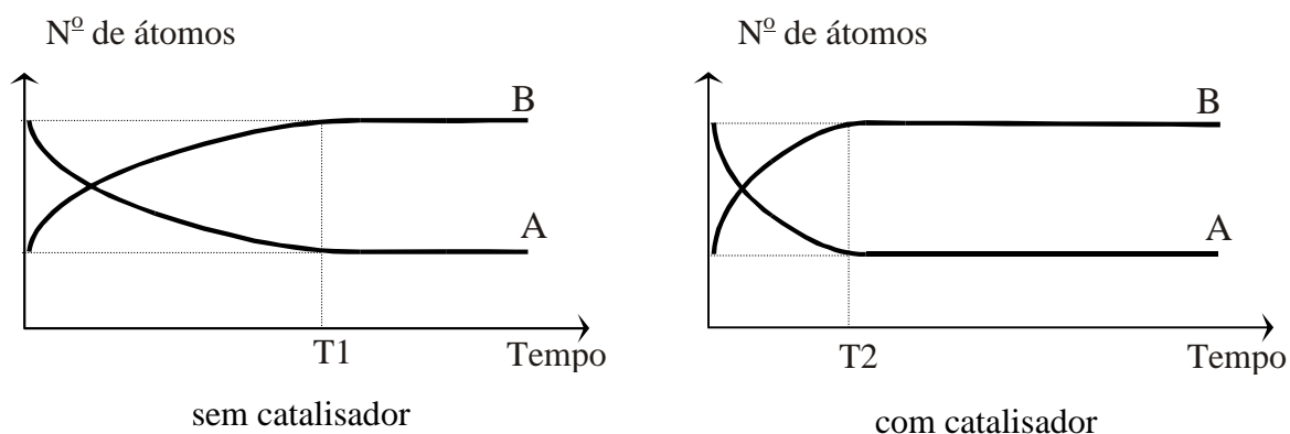
Figura 7. Representação esquemática do processo de uma reação hipotética, em função do tempo, sem e com a presença do catalisador.
