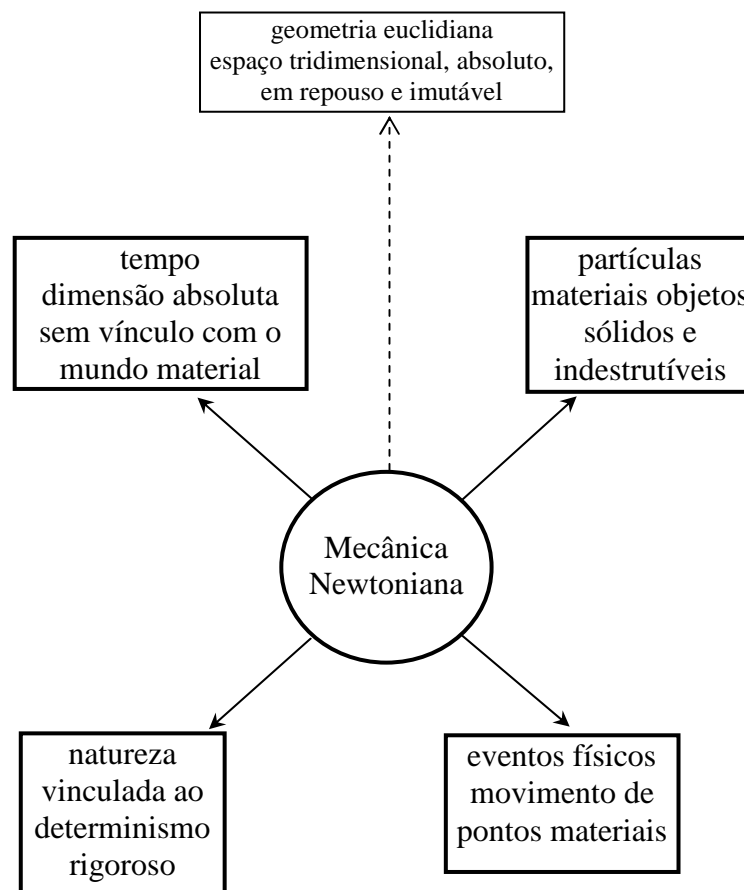
Figura 8. Resumo esquemático da Física Clássica.
