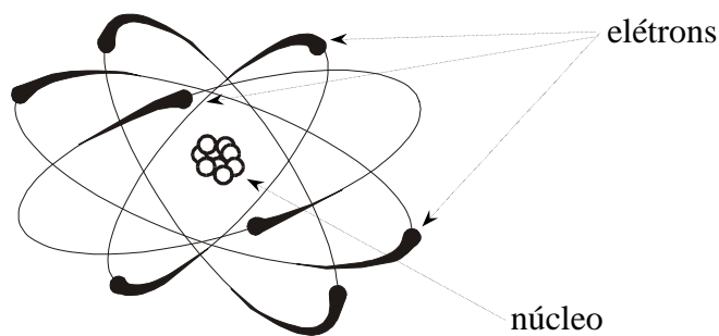
Figura 13. Representação do átomo como concebido por Bohr.
